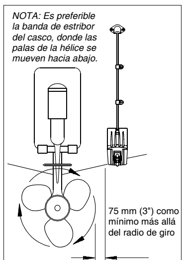
Figura 2. Ubicación para montaje en barcos de un solo motor
